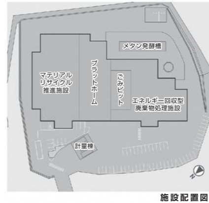
施設配置図
