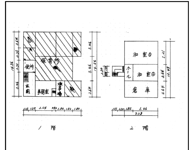
建物配置図
